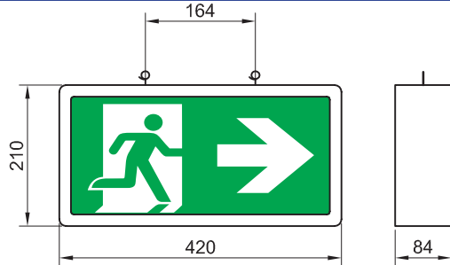
Kettenmontage (Universal)
