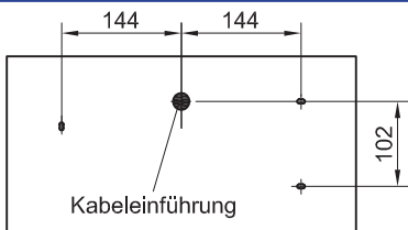
Bohrplan Wandblech
