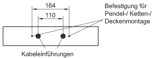
Lochabstände
