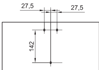
Bohrplan Universalmontage
