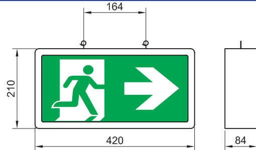
Kettenmontage (Universal)
