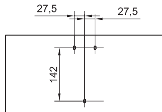
Bohrplan Universalmontage
